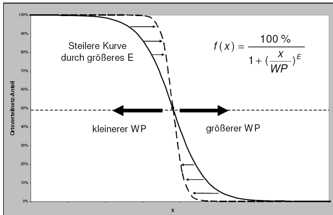
Abbildung 1: Abbildung der Sigmoidfunktion 1
